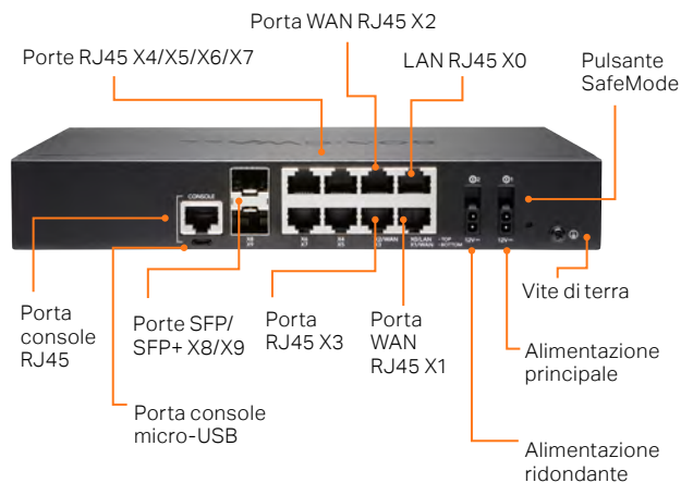
Pannello posteriore TZ670W
