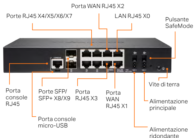
Pannello posteriore TZ570W
